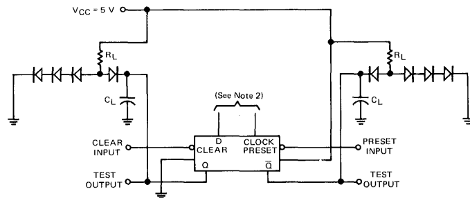
9N74/5474, 7474 TEST CIRCUIT
