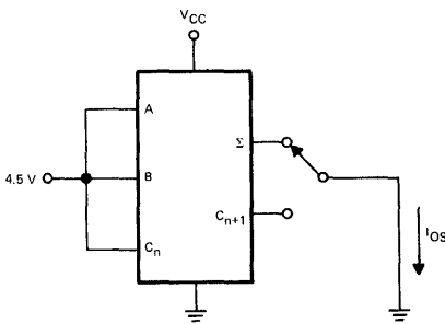
Fig. 4 - I_{OS}
