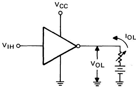
Fig. 65 V_{IH}, V_{OL}
