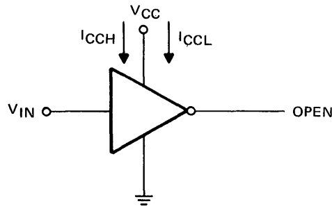
Fig. 69 I_{CCH}, I_{CCL}
