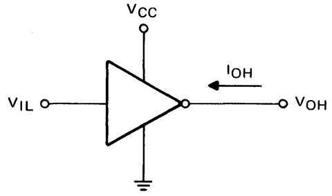
Fig. 66 V_{IL}, I_{OH}
