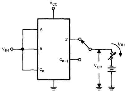
Fig. 1 - V_{IH}, V_{OH}
