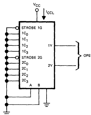
Fig. 5 I_{CCL}
