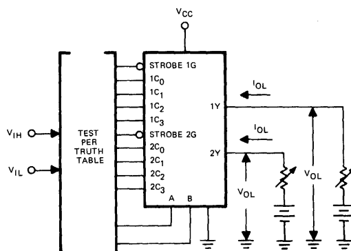
Fig. 2 V_{IH} , V_{IL} , V_{OL}
