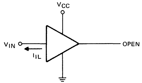
Fig. 73 I_{IL}
